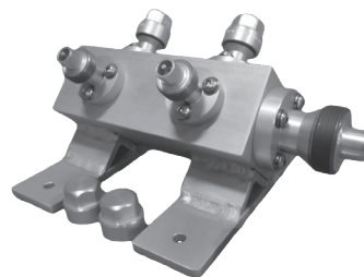
Colector de 4 puertos para cilindros D-240-R002 4 x DN8/1 x DN20
